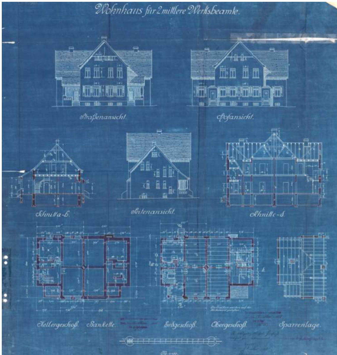
Bauzeichnung von 1915 Quelle: städtische Bauakten
